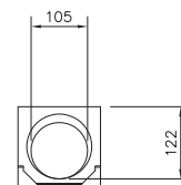
Canal SlimLine 50cm Registrable DN100 y DN150 Canal SlimLine 50cm Inspeção DN100 e DN150
