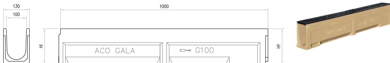
Canal Gala G100 - Canal Gala G100
