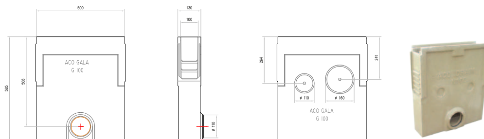
Sumidero Gala G100 - Sumidouro Gala G100
