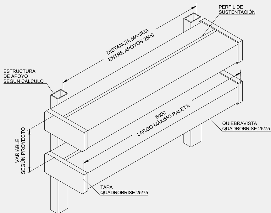
DETALLE QUADROBISE 25/75 DENTRO DE VANO
