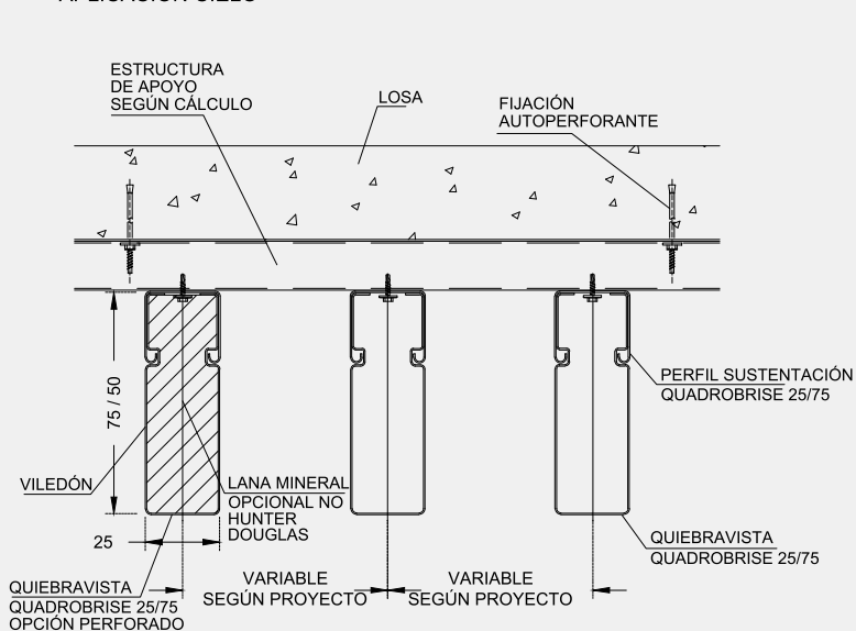
DETALLE QUADROBISE 25/75 APLICACION CIELO
